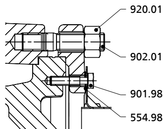
III. 24: Version avec fond de refoulement pincé
