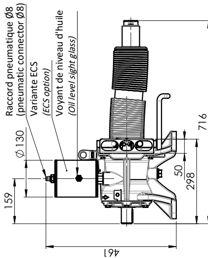
TRANSMISSION AVEC BMS et ECS (TRANSMISSION BLOCK WITH BMS & ECS) H FLO & G FLO 25
