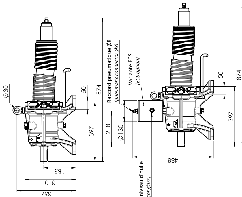
BMS monté à droite (BMS right mounted)
