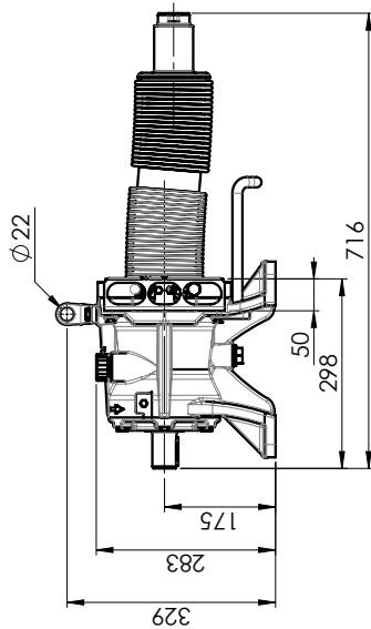
TRANSMISSION AVEC BMS et ECS (TRANSMISSION BLOCK WITH BMS & ECS) H FLO & G FLO 25
