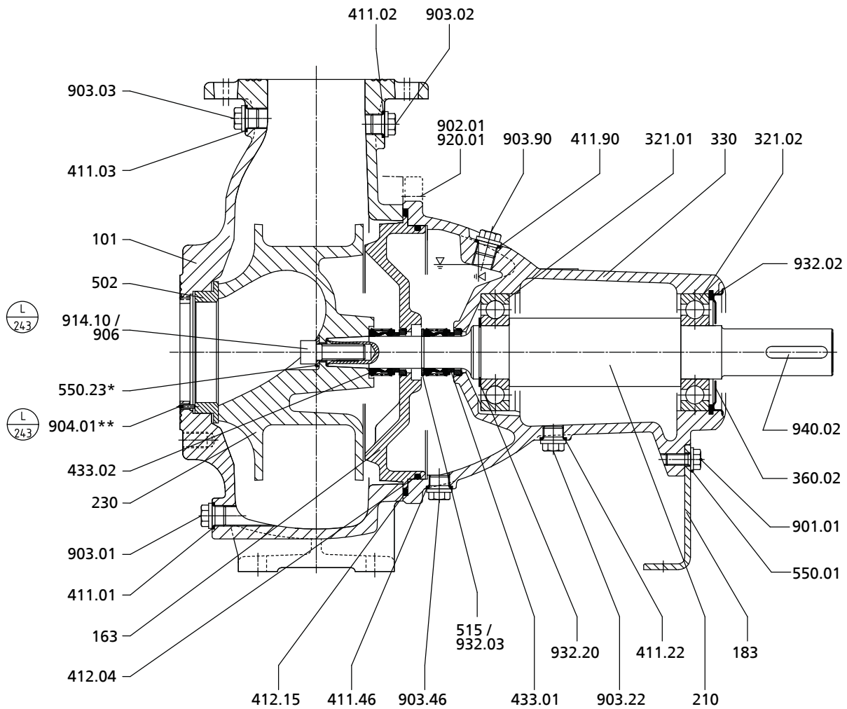
III. 1: Plan d'ensemble Sewatec - support de palier S01, S02, S03, S04 avec forme de roue E
